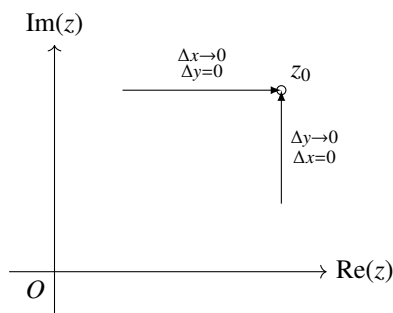
图 1.5: 逼近 z_0 的两种特殊方式.
